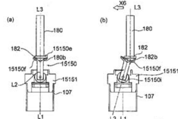
“万向节”齿轮结构
