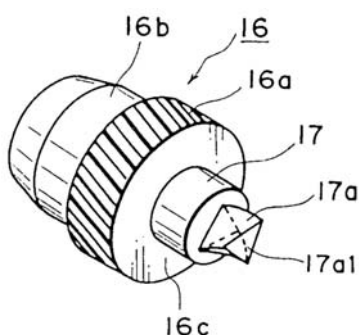
扭曲齿轮
