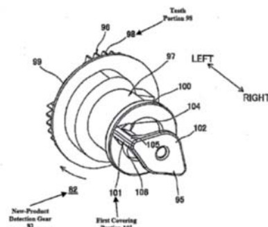
检测齿轮结构
